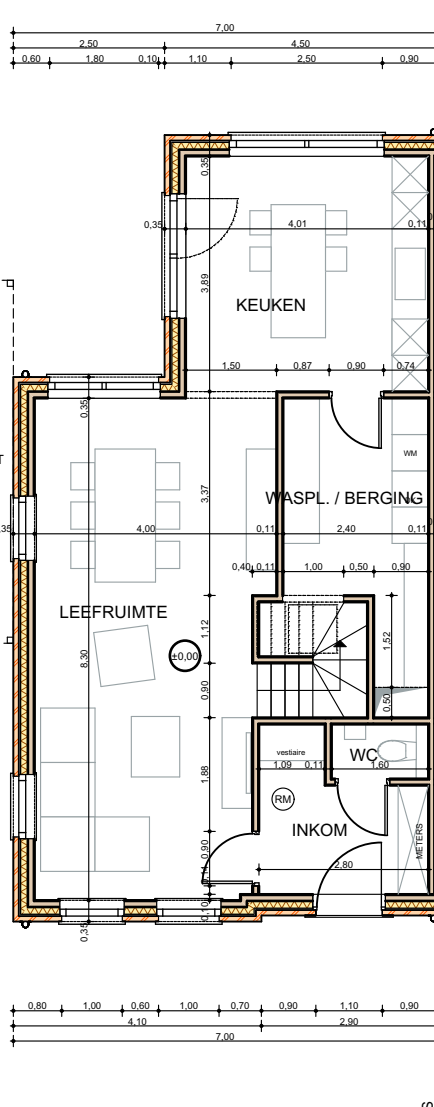
GRONDPLAN
