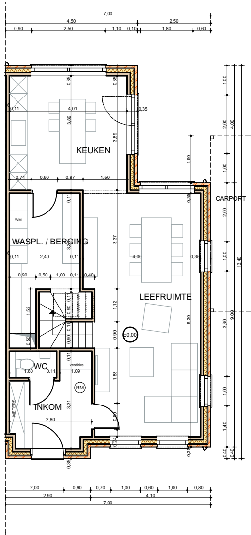
GRONDPLAN
