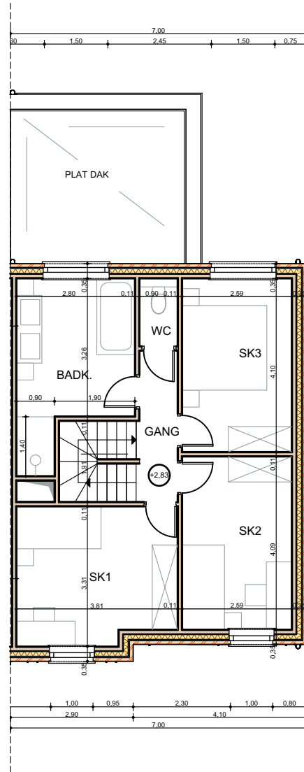
1e VERDIEPING
